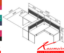
Modular MT-WS012 (ชุด workstation 2 ที่นั่ง) 3255(W) x 1655(D) x 1200(H) mm.
