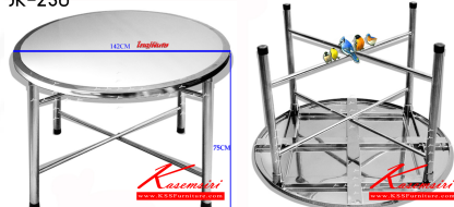
JK-230
