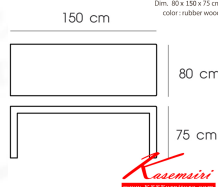
PN94126-Q150 Dim. 80 x 150 x 75 cm color : rubber wood
