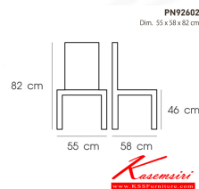
PN92602 Dim. 55 x 58 x 82 cm color : white
